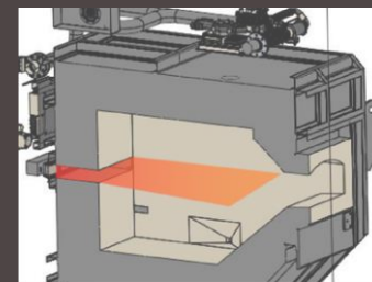
Warmhaltezone
